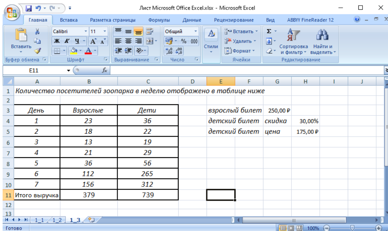
Рис. 3.3 – Лист Excel
