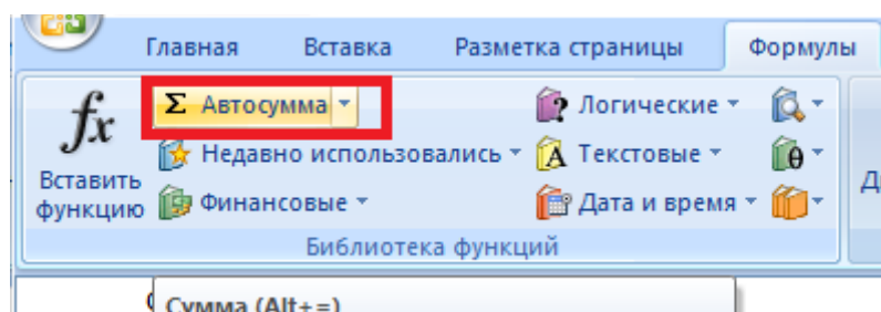
Рис. 3.2 – Формула Автосумма
