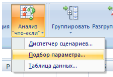
Рис. 7.2 – Подбор параметра
