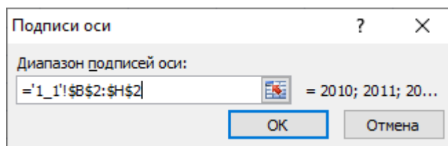
Рис. 1.5 – Подписи оси
