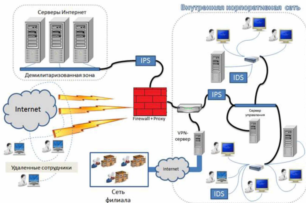
Рисунок 16–Диаграмма развертывания КИС
