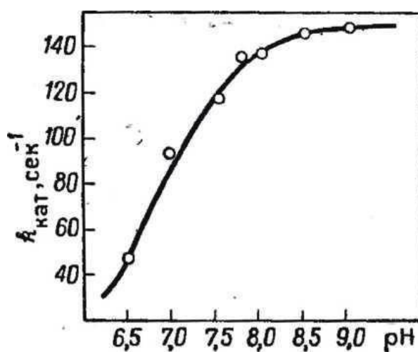
Рис. 5. pH-Зависимость каталитической константы скорости гидролиза этилового эфира N-ацетил-L-тирозина, катализируемого \alpha -химотрипсином
