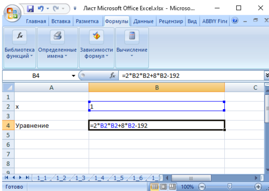
Рис. 8.1 – Подготовленный лист Excel
