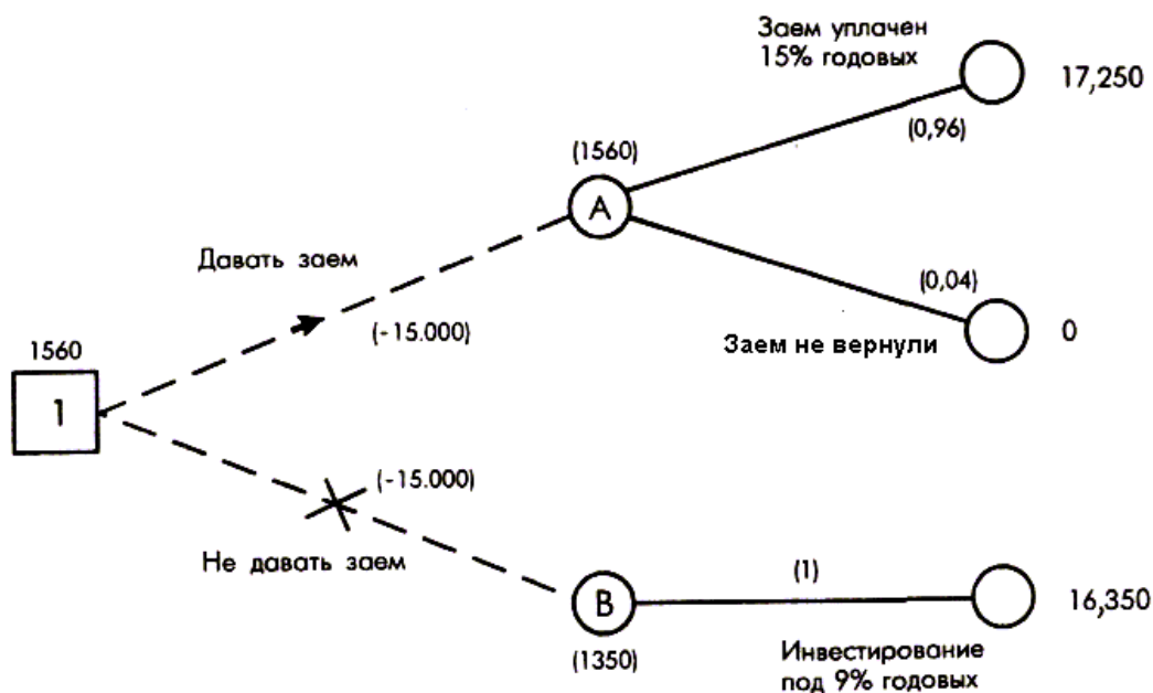
Рисунок 1 – «Дерево» решений
